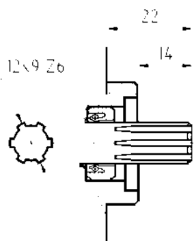
Coppia max 38 Nm Max torque 38 Nm
