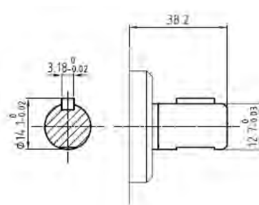
Coppia max 35 Nm Max torque 35 Nm
