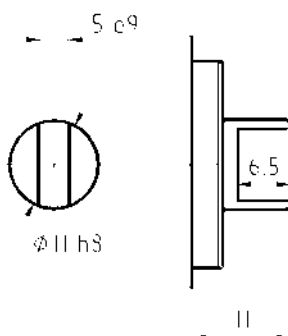
Coppia max 24 Nm Max torque 24 Nm
