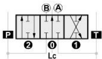
A-B dicht P-T rondpomp
